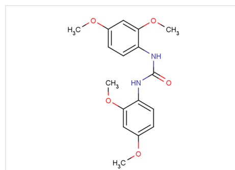
Structure Pygmaniline B, CAS 56402-79-0
