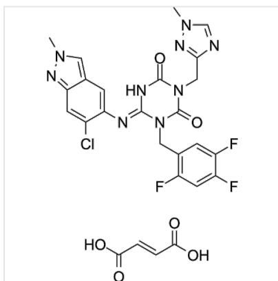
Structure Ensitrelvir fumarate, CAS 2757470-18-9
