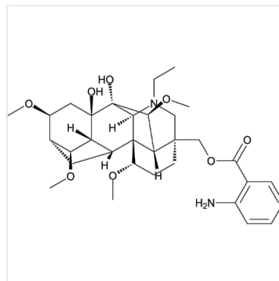
Structure Anthranolglycoctonine, CAS 22413-78-1
