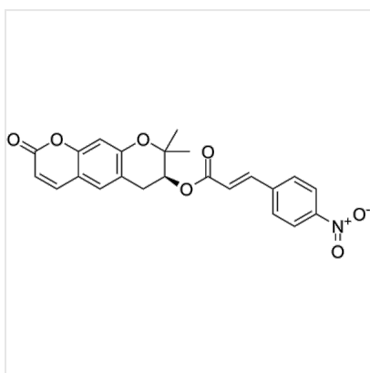
Structure LKY-047, CAS 1954681-29-8
