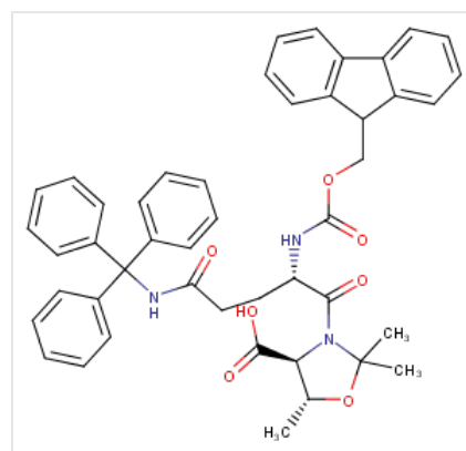
Structure Fmoc-Gln(Trt)-Thr(ψ(Me,Me)pro)-OH, CAS 1572725-72-4
