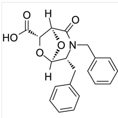
Structure Udonitrectag, CAS 1458063-04-1
