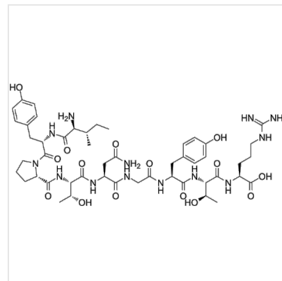
Structure IYPTNGYTR, CAS 1431957-72-0
