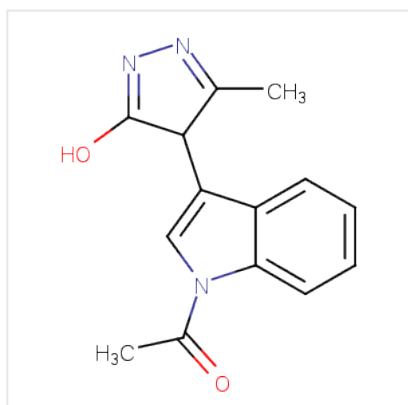
Structure SiA-IFN-1, CAS 300839-31-0
