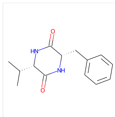
Structure Cyclo(L-Phe-L-Val), CAS 35590-86-4
