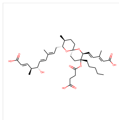
Structure Reveromycin D, CAS 144860-70-8
