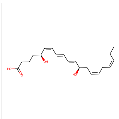
Structure Leukotriene B5, CAS 80445-66-5
